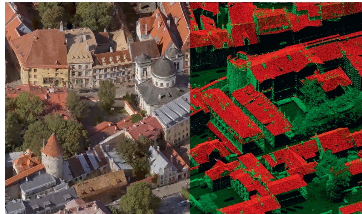
Vasemmalla Gaussian Splat –malli ja oikealla laserskannatut ja luokitellut pisteet
